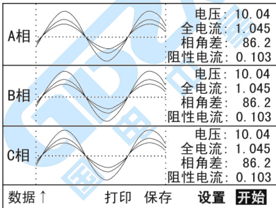
图 9 试验界面 1
