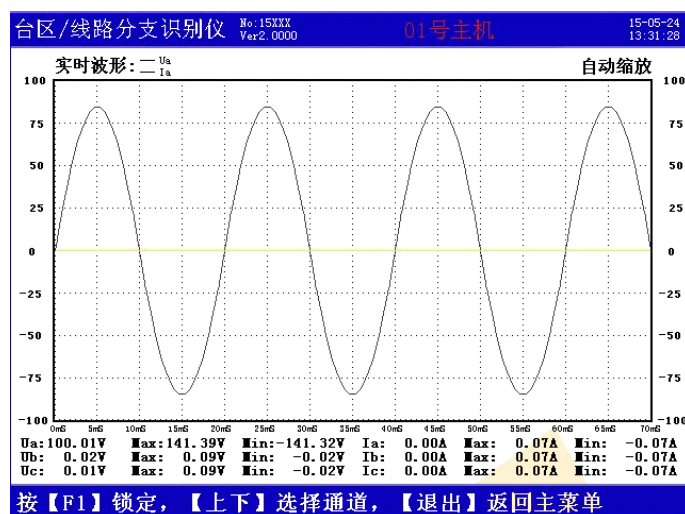
图 17 波形显示屏
