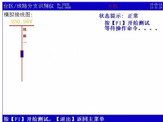
图 7 台区识别初始屏（分机）
