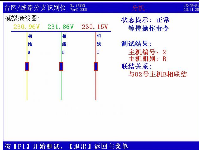
图 15 台变互测结果屏（分机）
