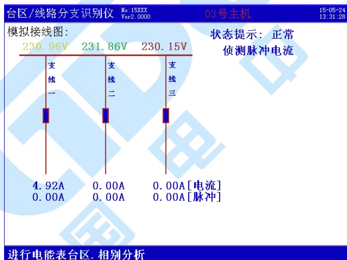
图 6 台区识别初始屏（主机）
