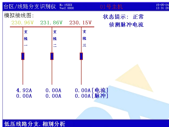
图 9 分支识别屏（主机）
