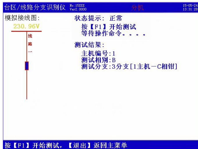
图 11 分支识别结果屏（分机）
