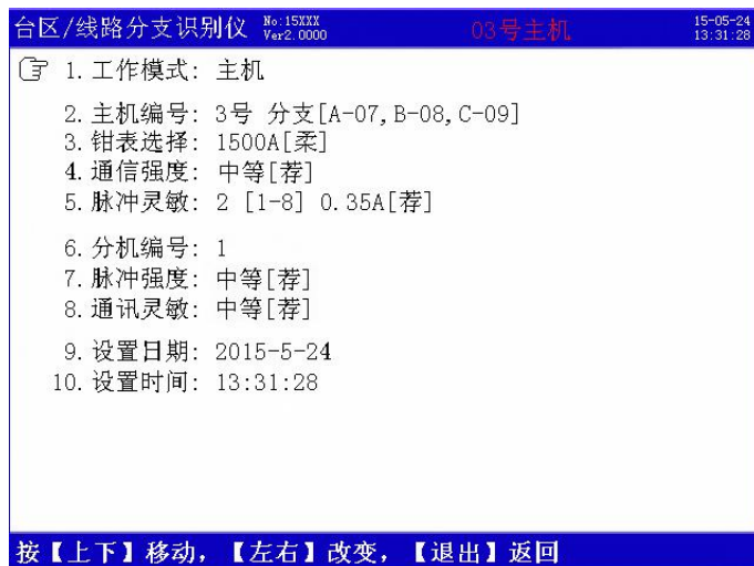
图 5 参数设置屏
