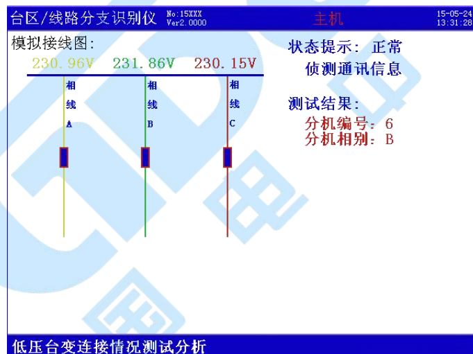
图 14 台变互测结果屏（主机）
