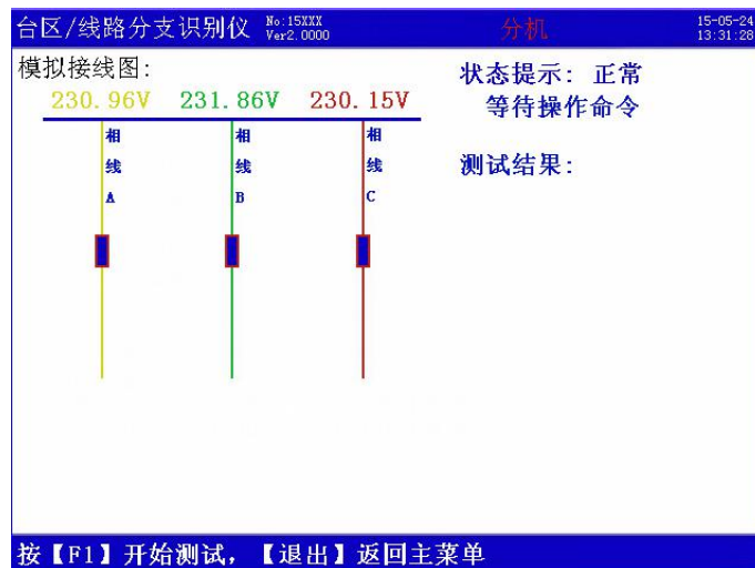
图 13 台变互测初始屏（分机）
