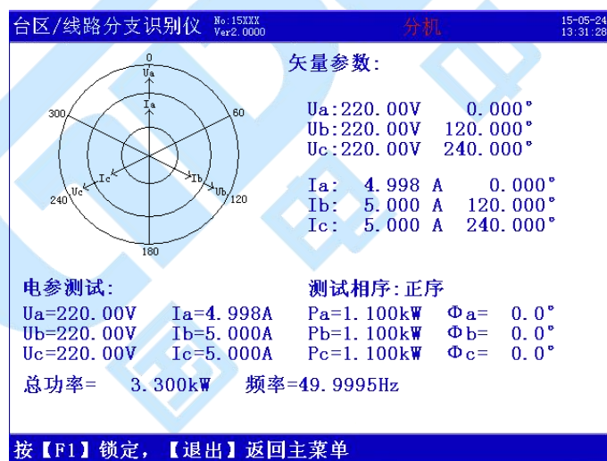
图 16 矢量电参屏
