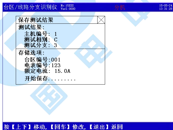
图 8 台区识别结果屏（分机）
