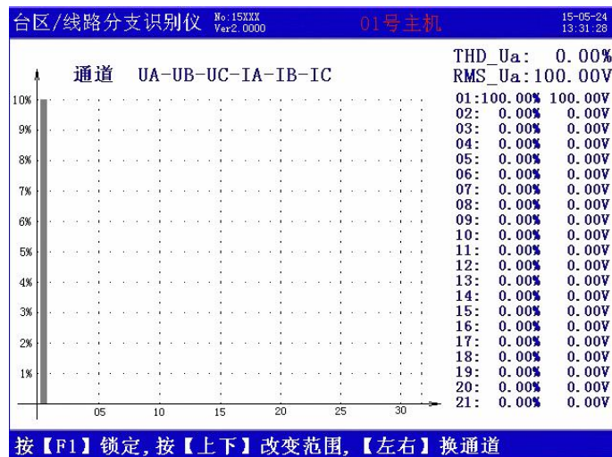
图 18 频谱分析屏
