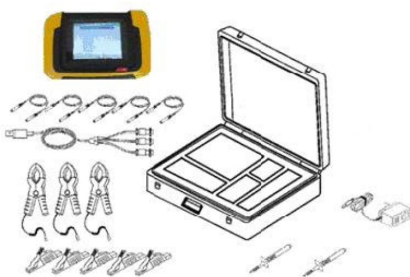
图 2-1 整机结构图（图中组件以实物为准）
