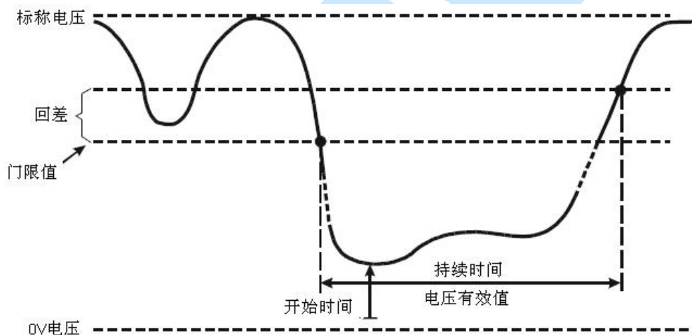
图 4-42 电压中断的特征
