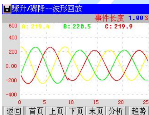
图 4-46 电压骤升/骤降波形记录
