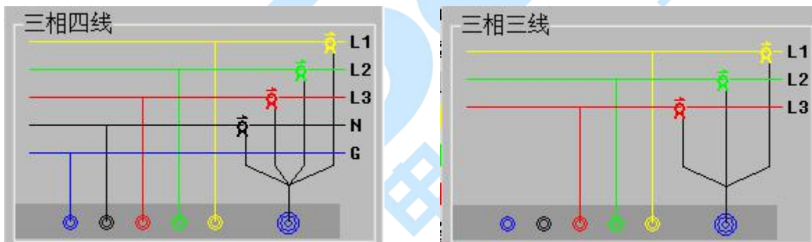
图 3-2 仪表测量连线示意图
