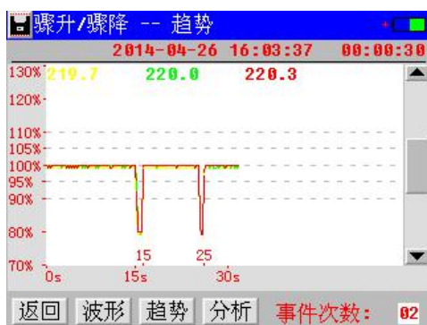
图 4-44(a) 电压骤降趋势图
