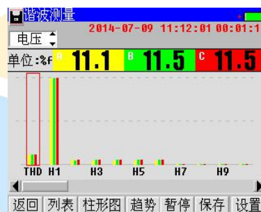
图 4-10 谐波柱型图
