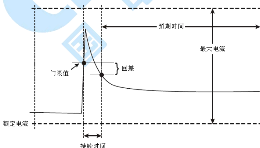
图 4-48 浪涌电流的特征
