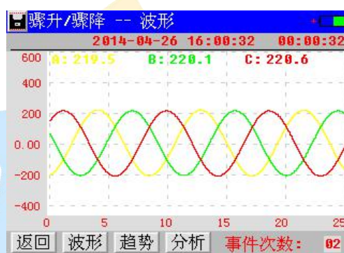
图 4-45 电压骤升/骤降波形显示
