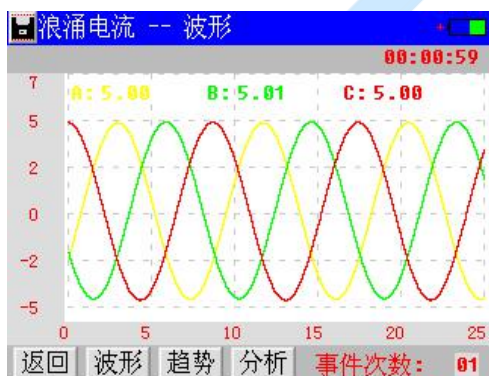
图 4-51 浪涌电流波形
