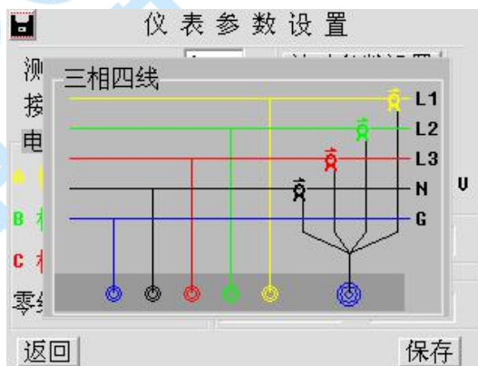
图 4-70(b) 接线图
