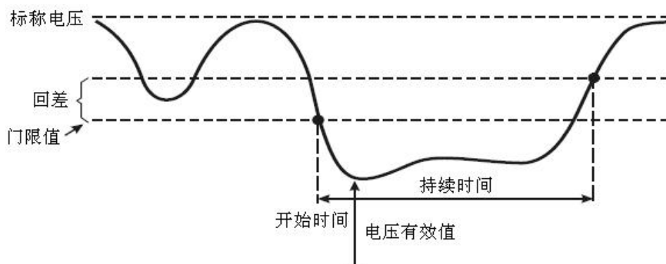
图 4-41 电压骤降的特征
