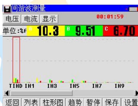
图 4-15 间谐波柱型图
