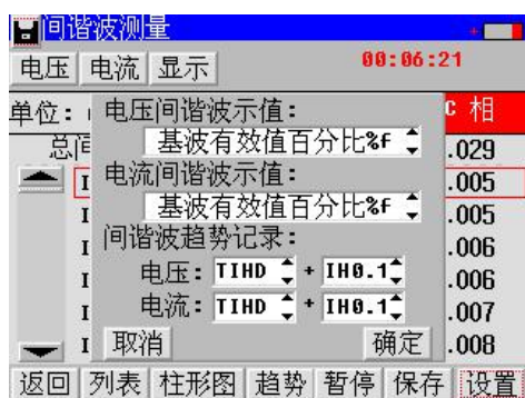
图 4-16 间谐波测量设置
