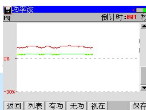
图 4-56(c) 无功显示
