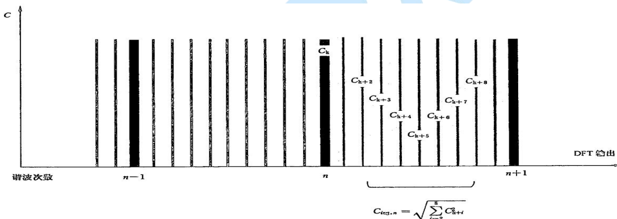
图 4-18 间谐波子集方均根值示意图 (50Hz 系统)
