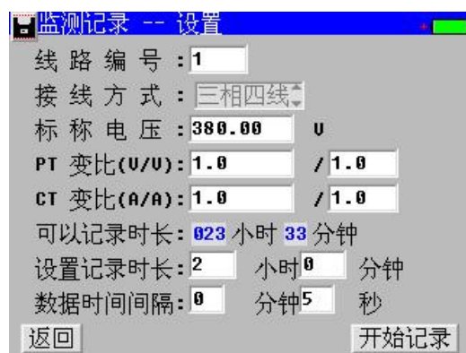
图 4-30 监测记录参数选择
