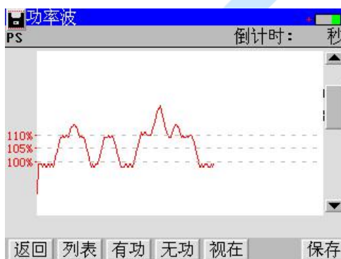
图 4-56(d) 视在显示
