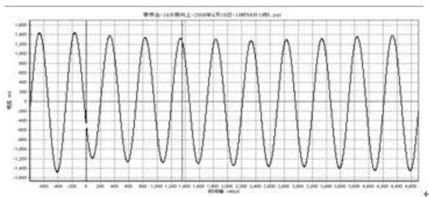
图A.4 三相三柱式变压器分接开关变换程序无异常交流零序试验波形 波形分析：三相三柱式变压器零序阻抗较小，分接开关切换过程中串入绕组的过渡电阻对试验电流限制作用比较明显，分接开关切换结束后零序电流逐步恢复稳定。
