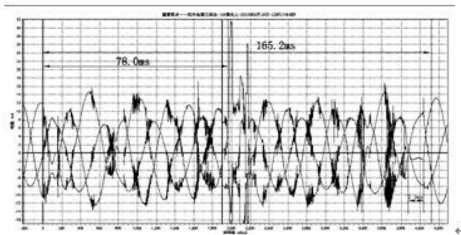
图A.12 双电阻V型分接开关极性开关触头不正 800 V三相交流试验波形
