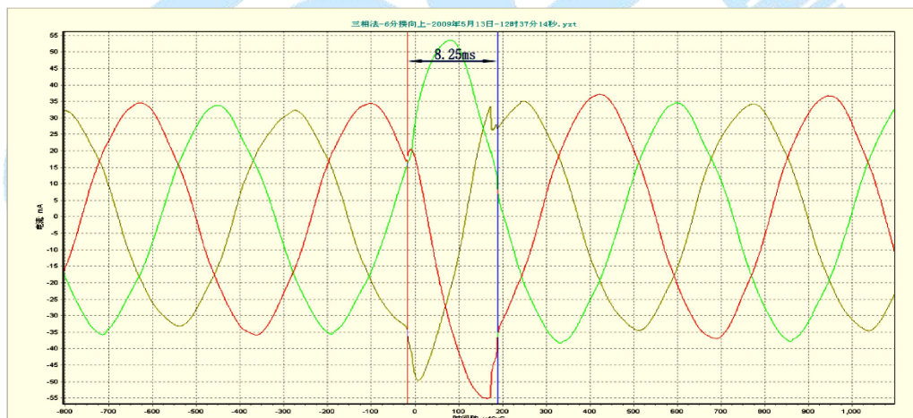
(图十一 B) 一次绕组 D 结线(8) 测试三相开断不同步时间
