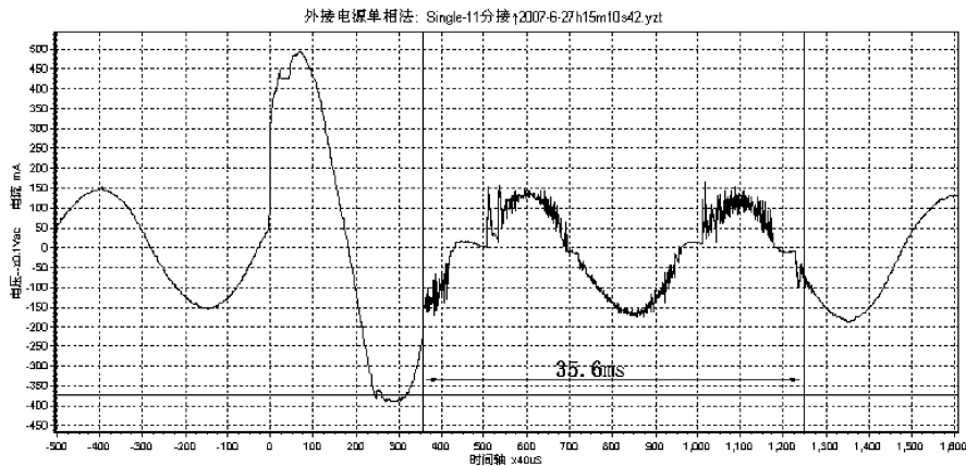
图A.11 双电阻V型分接开关过渡触头接触不良单相交流 6 400 V试验波形
