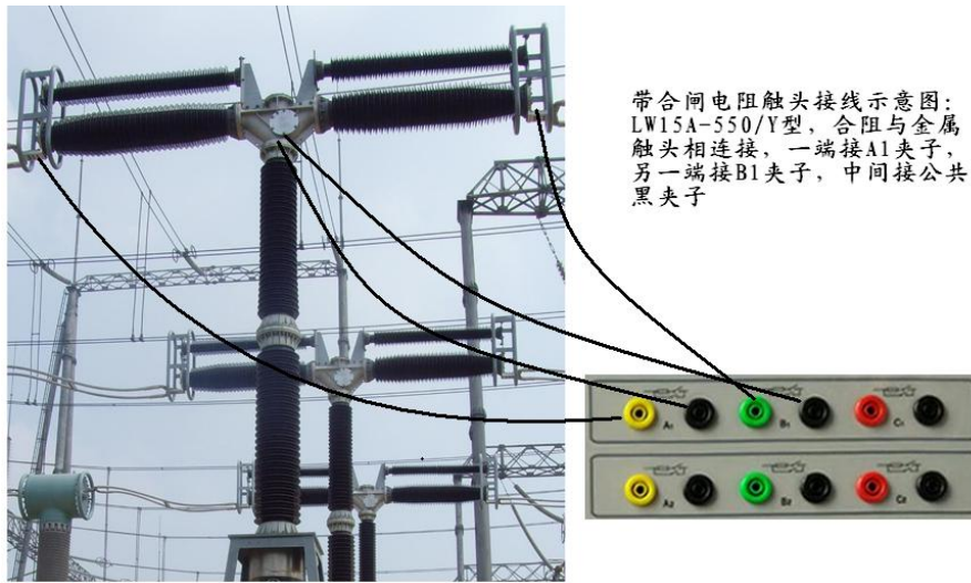
合闸电阻接线示意图
