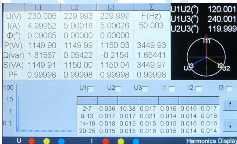
图 11 谐波显示
