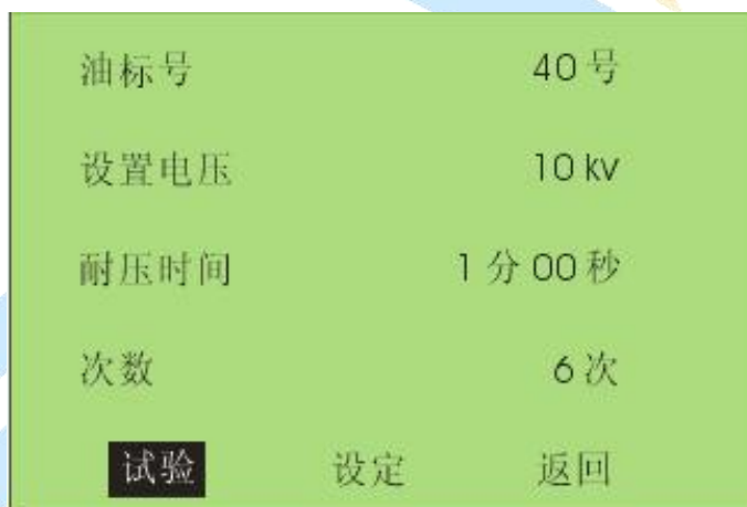
图 5.5 耐压试验主界面
