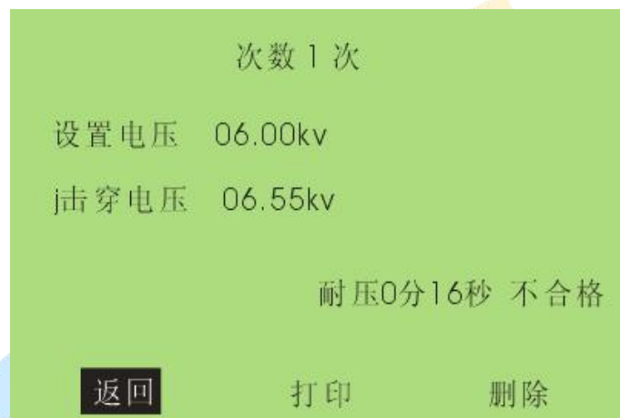
图 5.9 耐压试验历史数据
