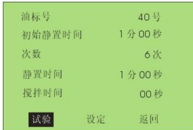
图 5.2 击穿试验主界面
