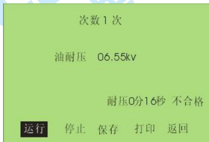
图 5.6 油耐压试验完成界面
