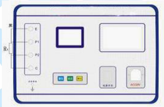
图 4 仪器自检原理接线图
