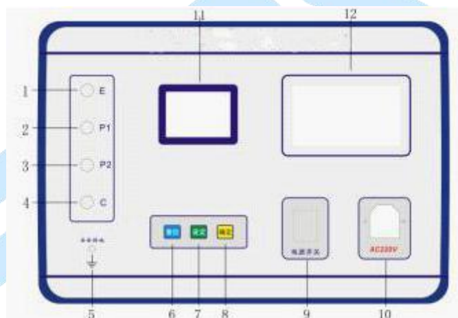
仪器面板布置图
