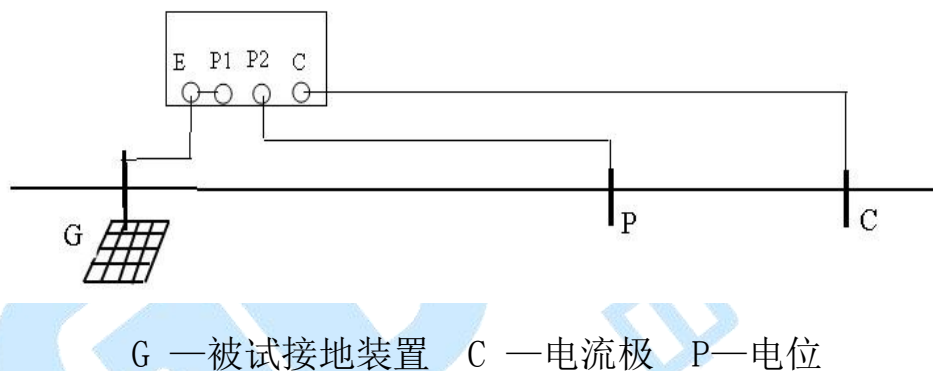
图 2 接地电阻测试接线示意图
