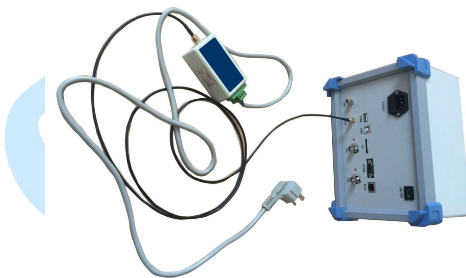
图 4-26 外同步接线图
