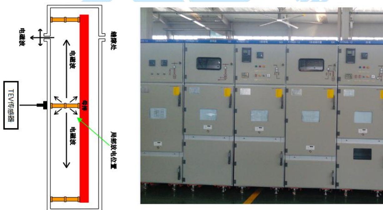
图 5-1 TEV 检测原理
