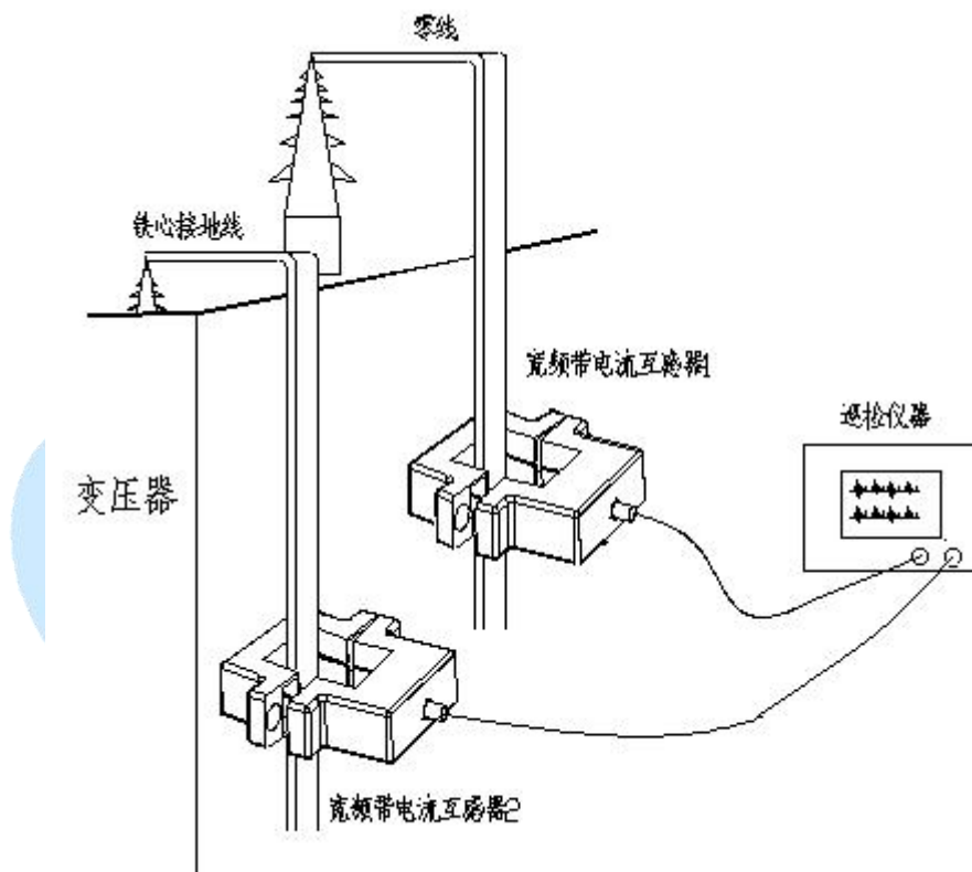
图 7-3 HFCT 检测位置
