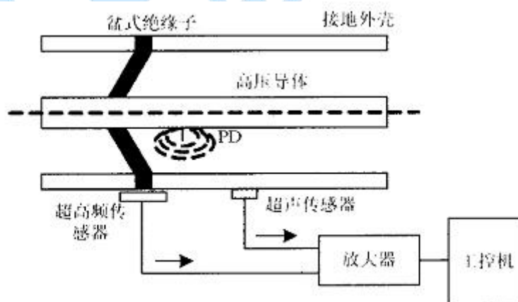
图 6-3 UHF 和超声波联合检测
