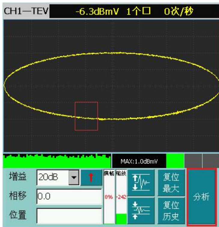
图 4- 16 开相位窗并进行单脉冲分析
