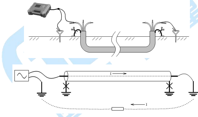
图 3-1-1 芯线 - 大地接线法
