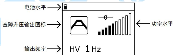
图 6-1-2 发射机查障升压输出界面
