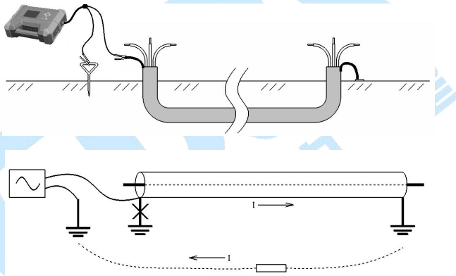
图 3-1-2 护层 - 大地接线法
