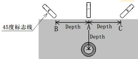
图 4-4-3 音谷 45°法测深
