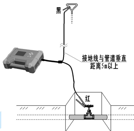
图 2-1-2 直连接线
