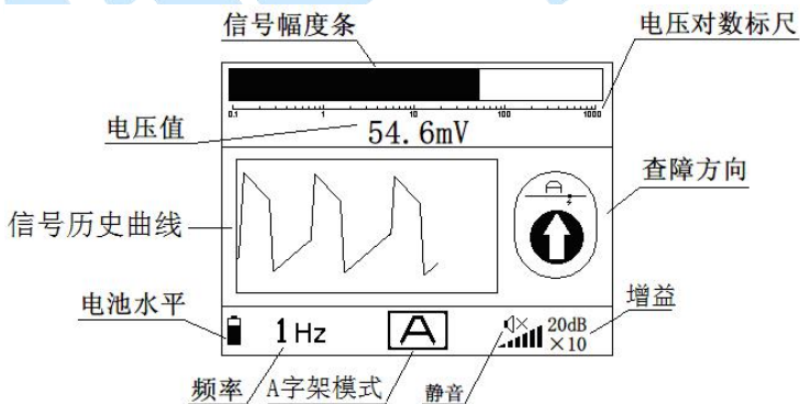
图 6-1-5 接收机 A 字架查障界面
