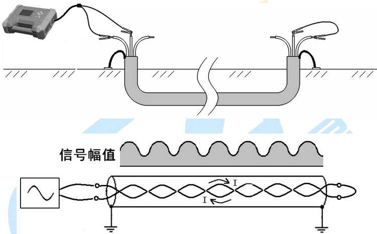
图 3-1-5 相间接法
