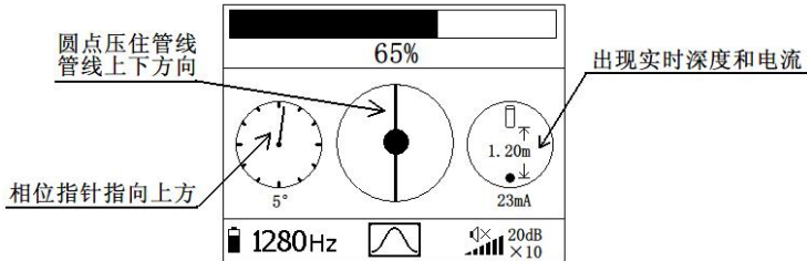
图 4-4-1 实时深度和电流测量
