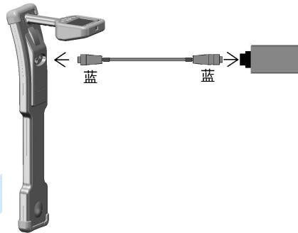
图 5-3-1 听诊器连接
