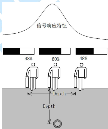
图 4-4-4 宽峰 80%法测深
