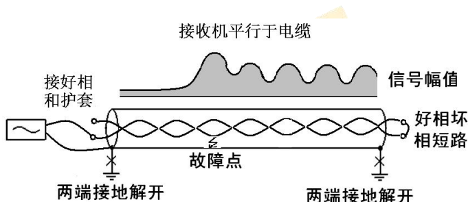
图7-2-1 相对铠装接地故障定点
