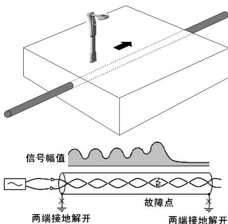
图 7-1-1 相间短路故障定点
