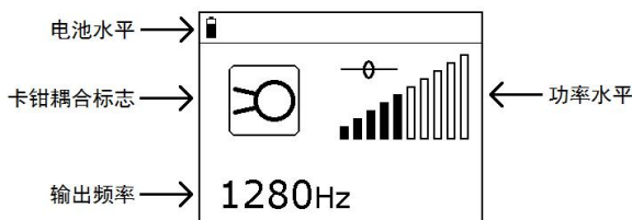
图 2-2-3 卡钳耦合输出界面显示
