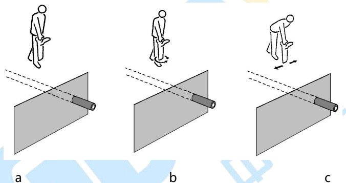
图 4-3-1 精确定位
