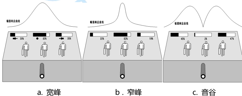
图 4-1-3 不同模式下的信号响应
