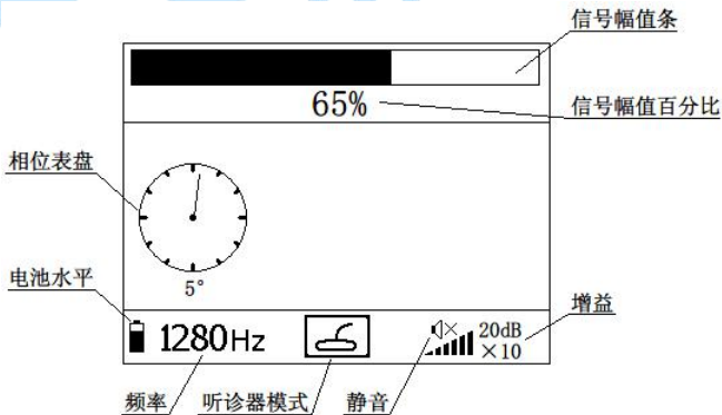
图 5-3-2 听诊器界面
