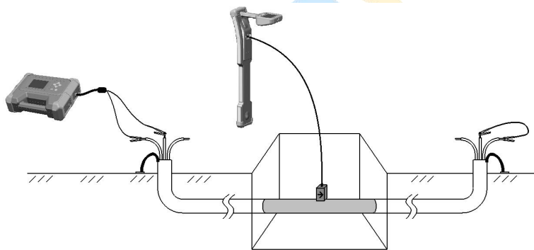
图 5-3-3 听诊器鉴别
