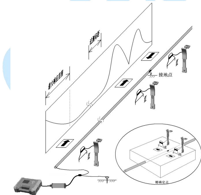
图 6-1-6 A 字架查障过程
