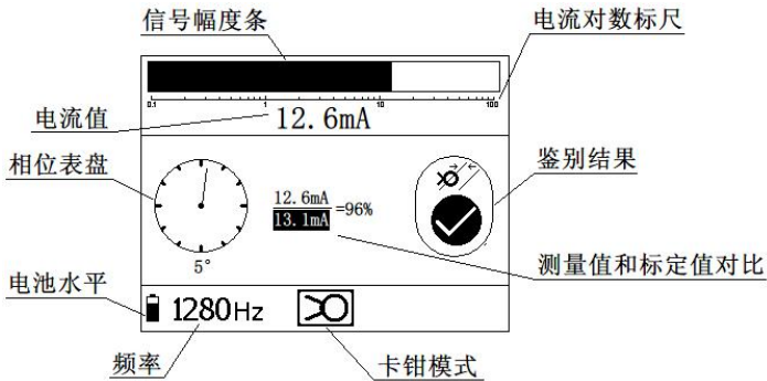
图 5-1-2 柔性卡钳鉴别界面
