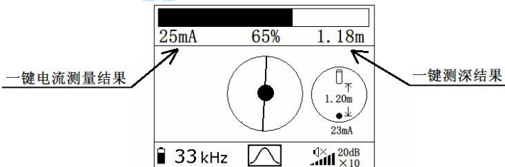
图 4-4-2 一键深度和电流测量
