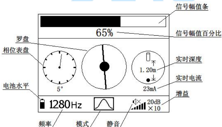
图 4-1-1 管线探测界面
