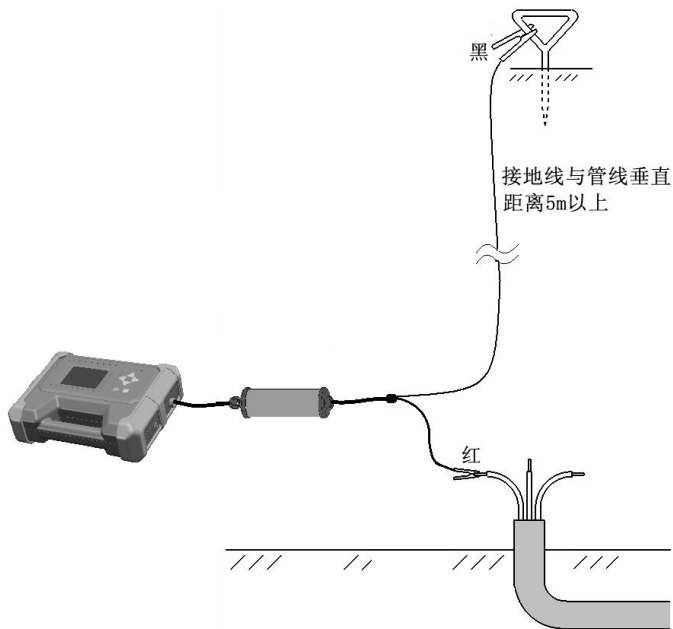
图 6-1-3 接地故障定点接线
