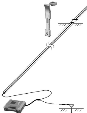
图7-3-1 断线故障接线
