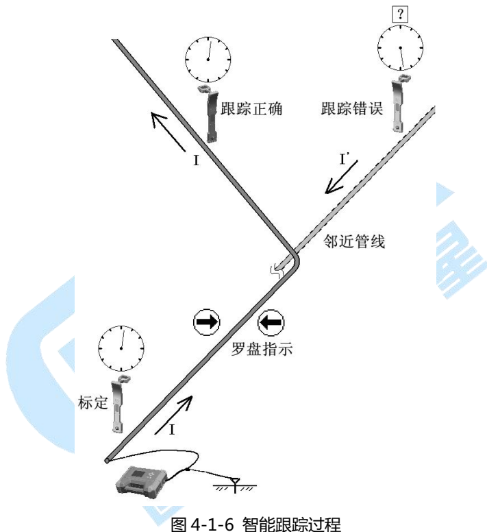
图 4-1-6 智能跟踪过程
