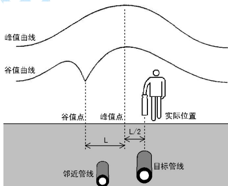
图 4-3-2 定位修正
