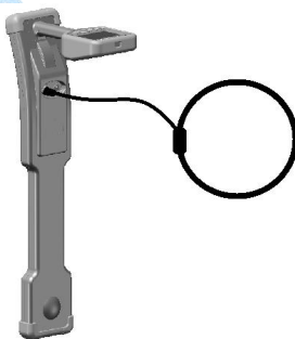
图 5-1-1 接收柔性卡钳连接
