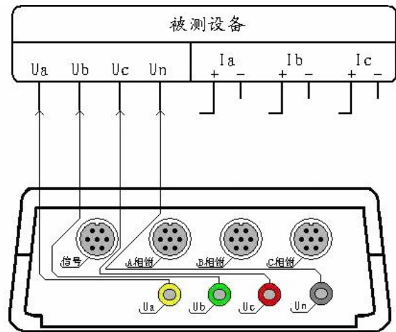
电压谐波测试接线图
