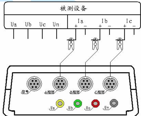
电流谐波测试接线图
