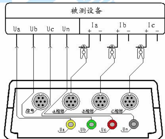
三相四线制设备测试接线图
