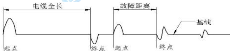
图（21） 故障点二次击穿测试波形
