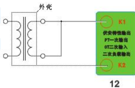
7. 接线图：图 7 (二次负载接线图)
