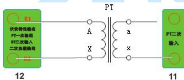
6. 接线图：图 6 (二次耐压接线图)
