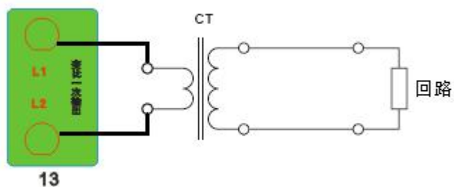
4. 接线图：图 4 (PT 伏安接线图)
