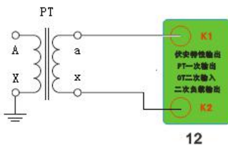
5. 接线图：图 5 (PT 变比接线图)
