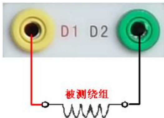
图 26 直阻测试接线图
