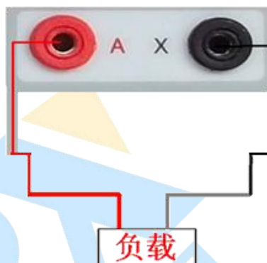
图 23 CT 二次负荷接线图
