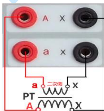
图 31 PT 变比极性 (角差比差) 接线图
