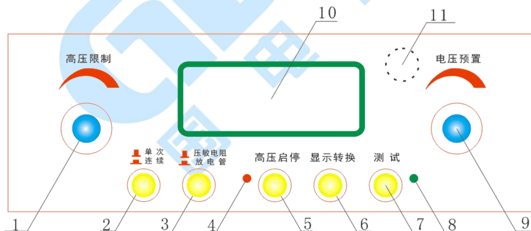
前面板图
