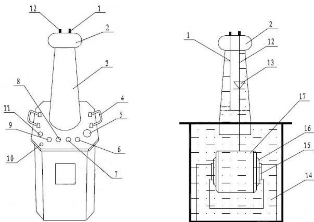
图1：单台工频耐压试验成套装置外部结构图
