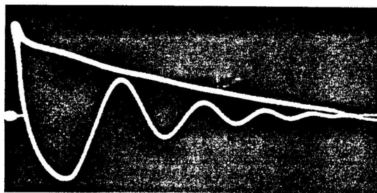
图 4—6 断线波形
