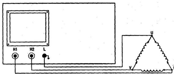
图 4-3 Δ（角）接法
