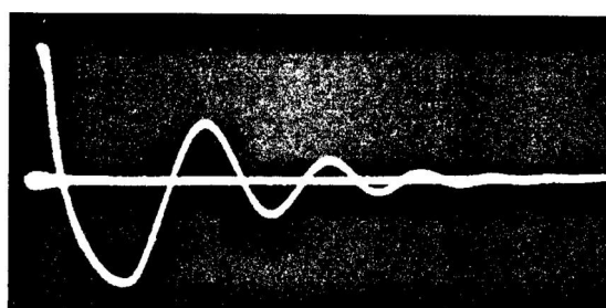
图 4-7 短路波形
