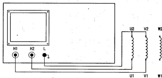
图 4-1 Φ（相）接法
