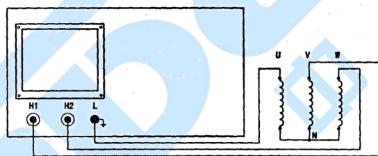
图 4—2 Y（线）接法
