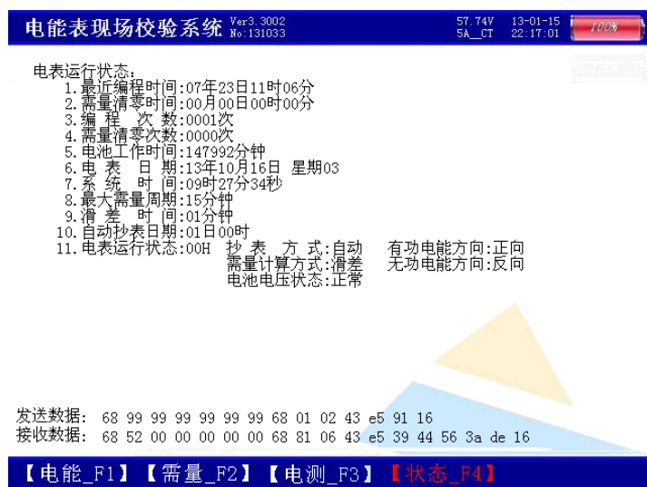
图 14 测试-485 状态
