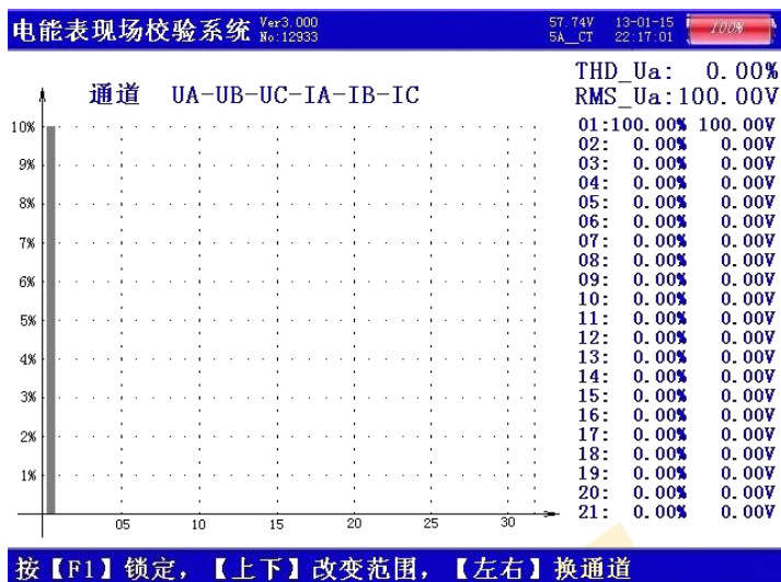
图 16 频谱分析屏
