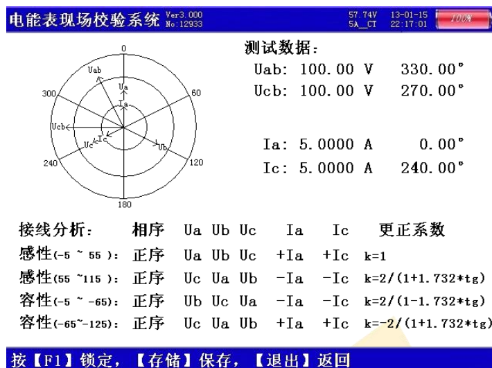
图 9 矢量分析屏—三相三线
