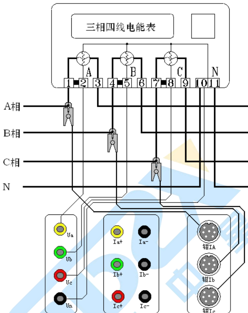
图 21 三相四线钳表接入测试
