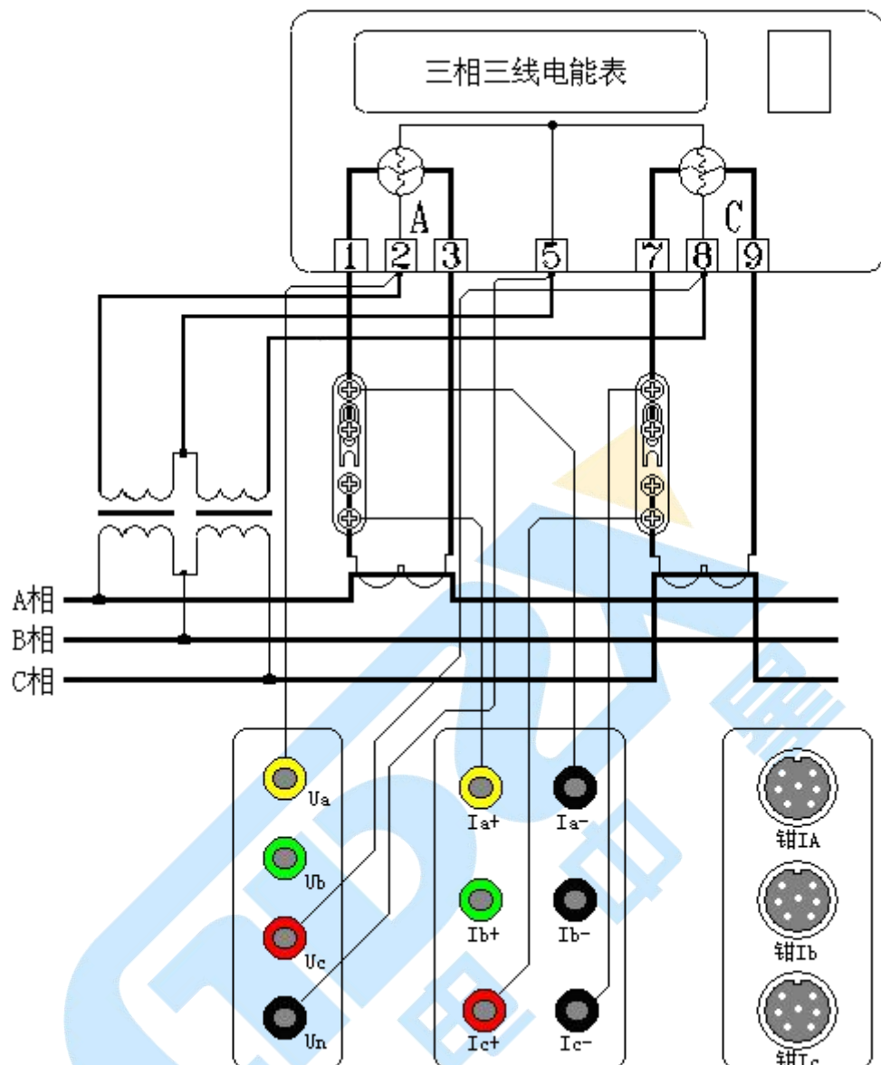
图 24 三相三线高压计量表计直接接入测试
