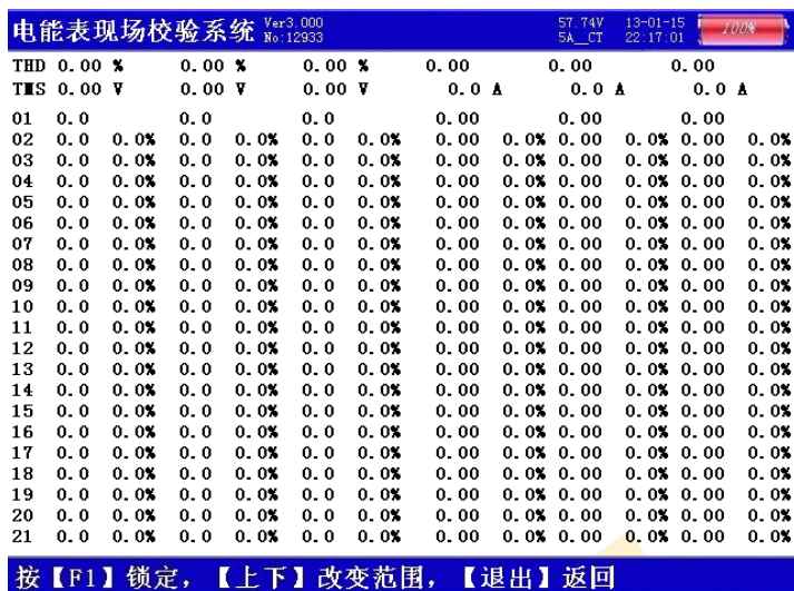
图 17 谐波测试屏
