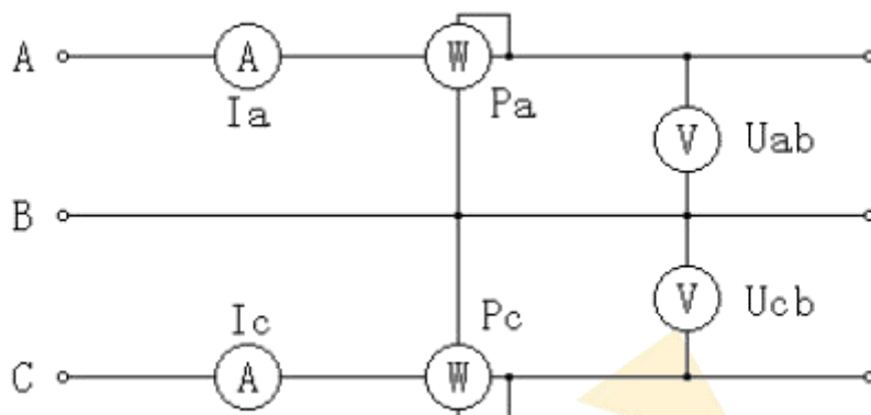
图 19 三相三线计量原理图
