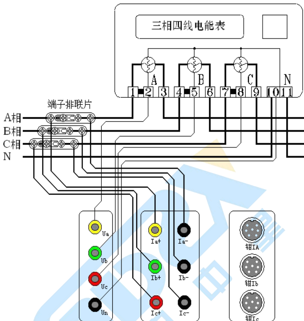
图 22 三相四线直接接入测试
