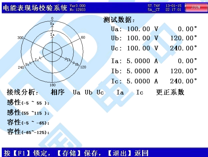
图 8 矢量分析屏—三相四线
