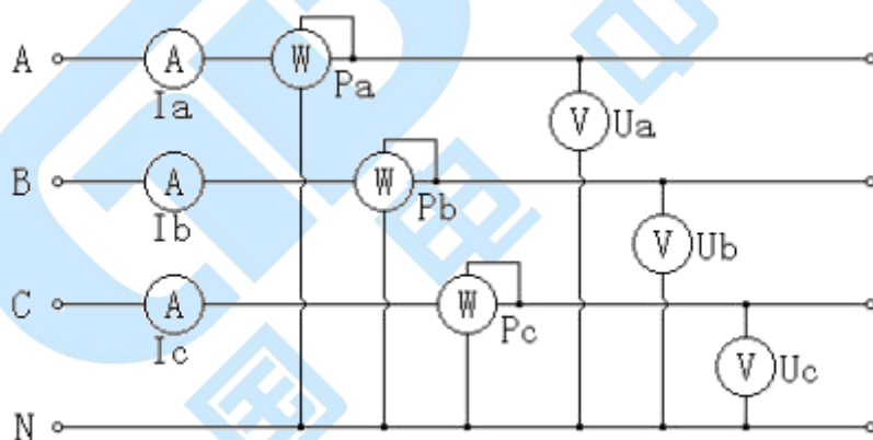
图 20 三相四线计量原理图
