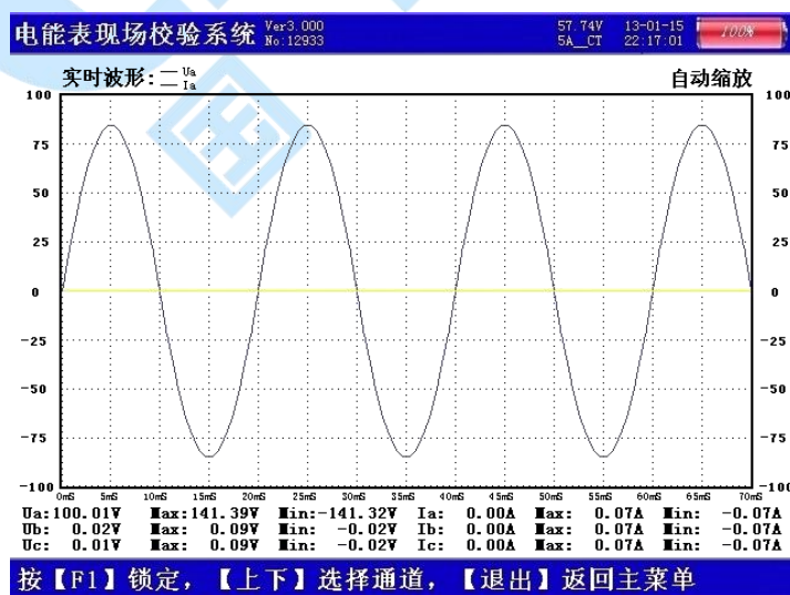
图 15 波形显示屏
