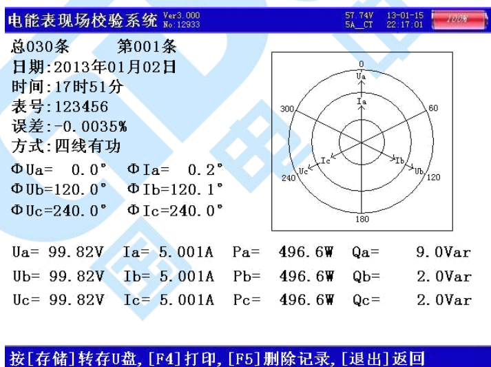
图 18 历史数据屏
