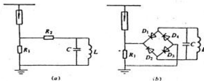
图 1 JS 型动作计数器的原理接线
