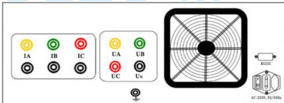
图 2 后面板图
