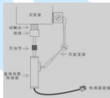
安装示意图
